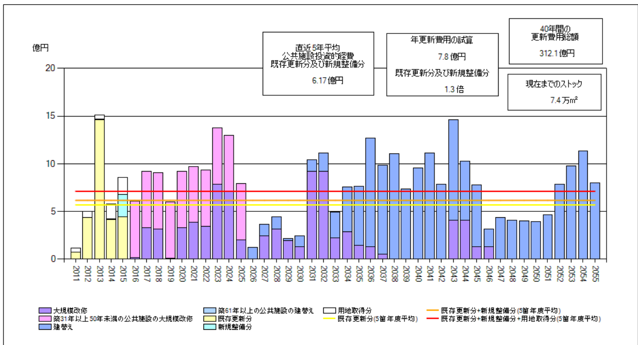
図表 2-12 公共施設の将来更新費用推計
