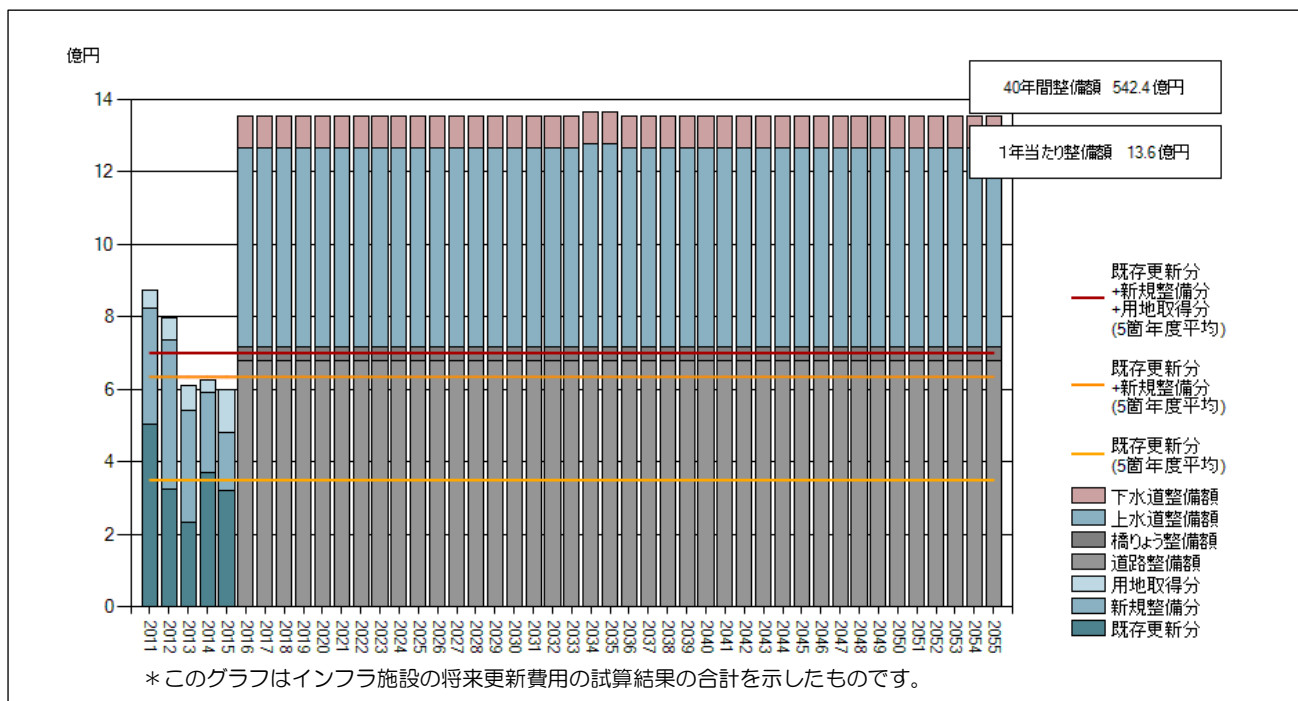
図表 2-14 インフラ施設の将来更新費用推計
