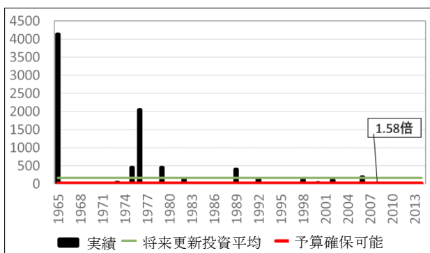
図表 4-4 建設年別橋りょう面積 (東洋大学 PPP 研究センター作成資料)
