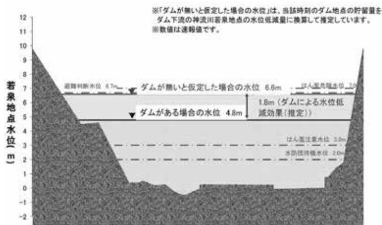
▲若泉地点(下久保ダム下流約9.5km)水位低減効果
